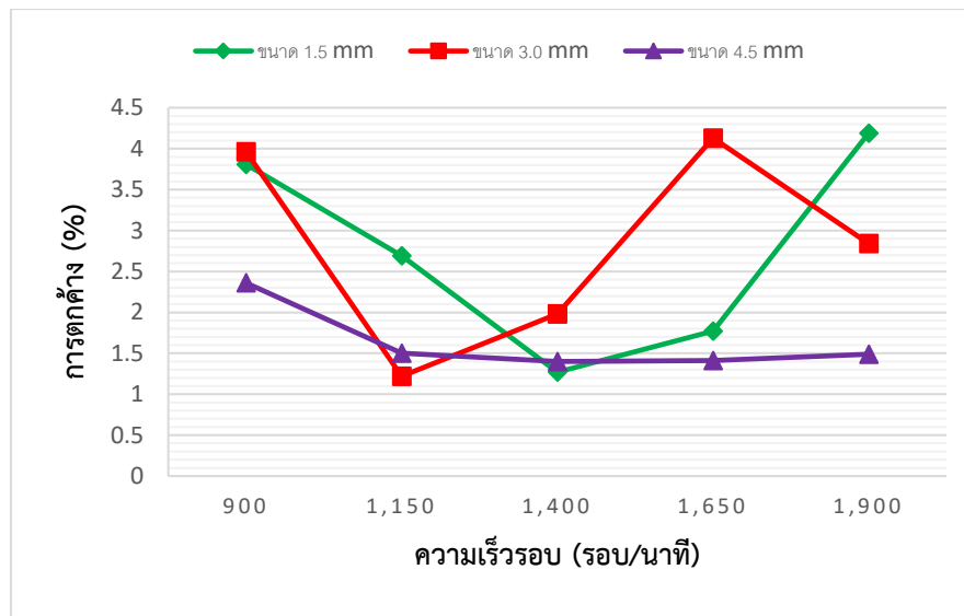
ภาพที่ 43 ผลการเปรียบเทียบของความเร็วรอบการกะเทาะและขนาดตะแกรงต่อการตกค้าง
