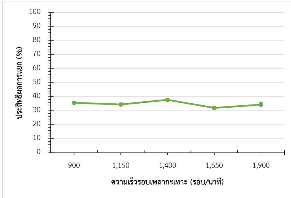
ภาพที่ 37 ผลของความเร็วรอบการกะเทาะต่อประสิทธิภาพการแยก
